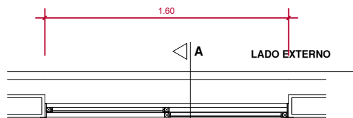
JA2 - PLANTA ESCALA 1:25
