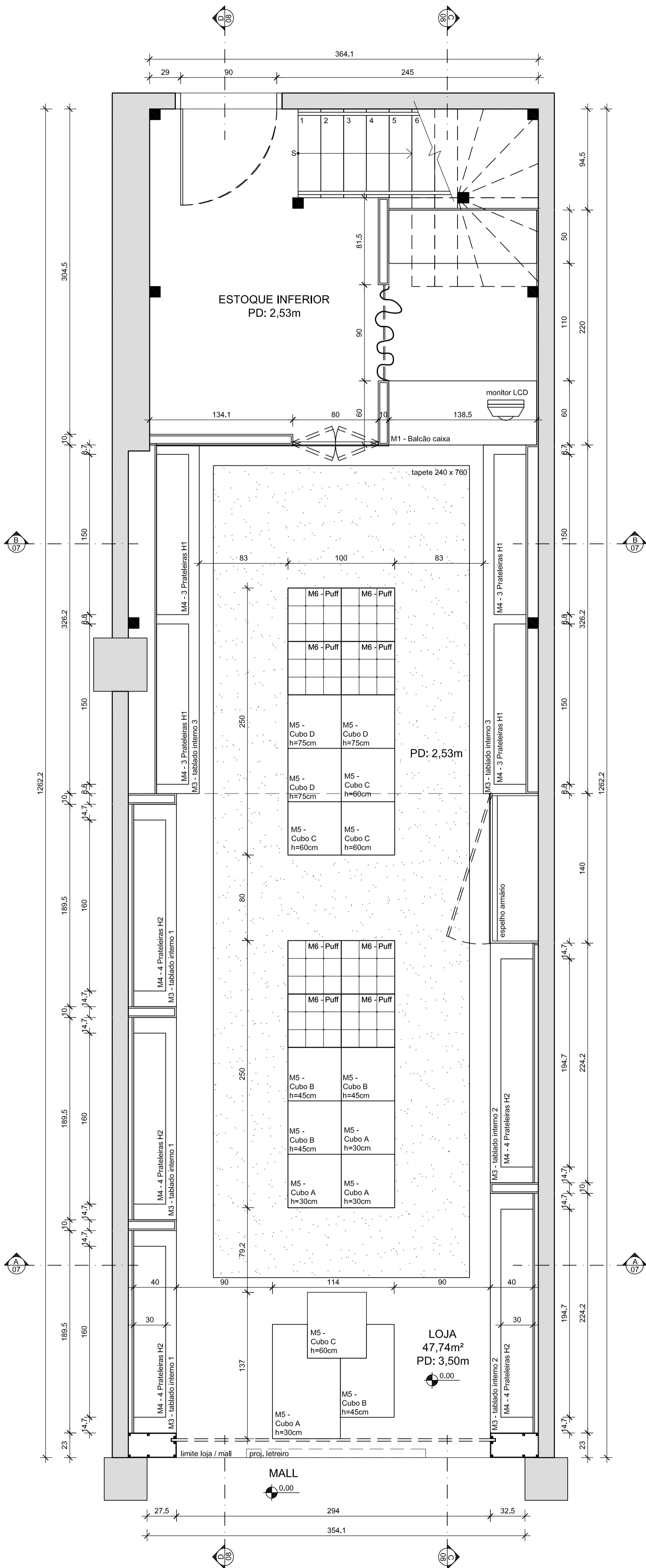
1 Planta baixa ESCALA: 1:25
